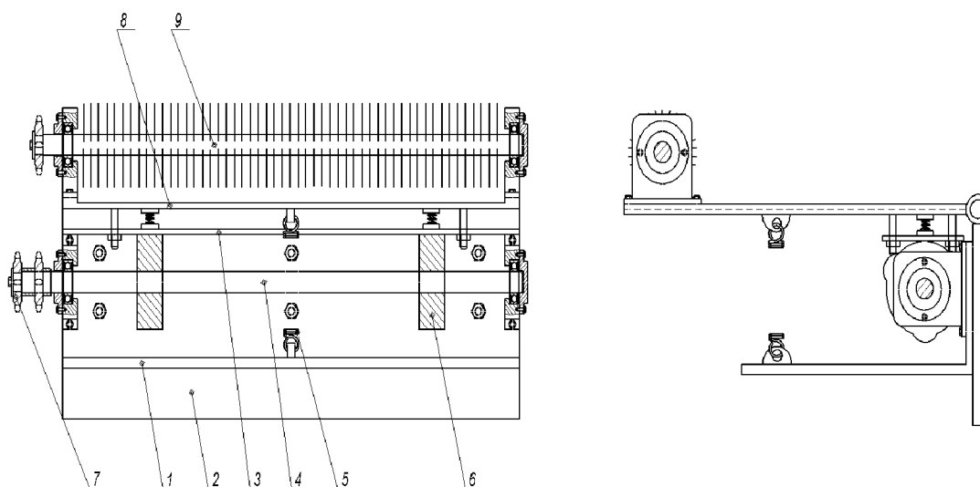
Рис. 1. Вибрационный высевальный аппарат
