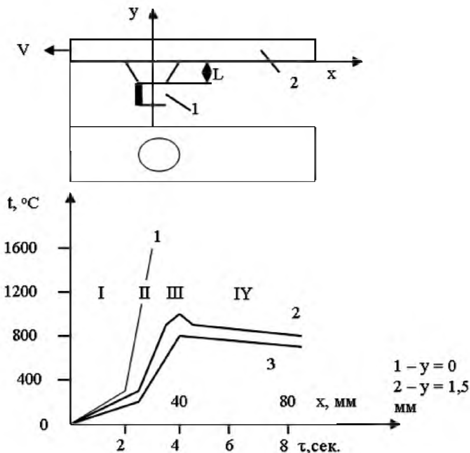
Рис.6. Схема экспериментальной установки и кривые нагрева
