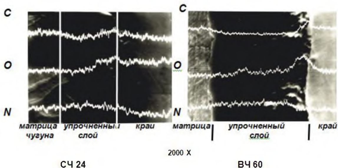
Рис.4. Распределение N, С и О по глубине карбонитрированного слоя
