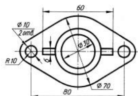
Деталь «крышка»
