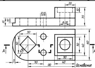
Деталь «основание»
