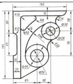
Контур детали «крюшка»
