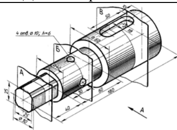
Деталь «вал»
