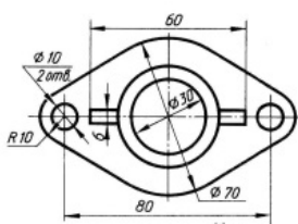
Деталь «крышка»
