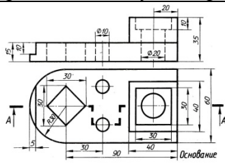
Деталь «основание»
