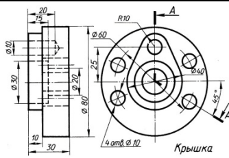
Деталь «крышка»
