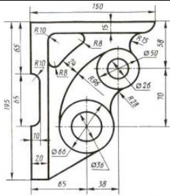
Контур детали «крышка»
