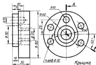
Рисунок 7 – Деталь «крышка»
