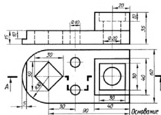
Рисунок 6 – Деталь «основание»
