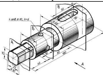
Деталь «вал»
