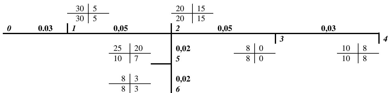
Расчетная схема сети вариант №1
