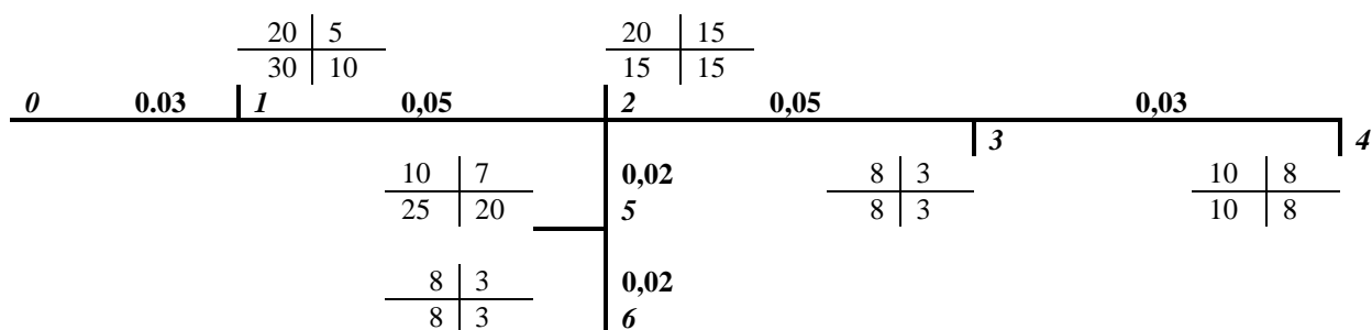
Расчетная схема сети вариант №2
