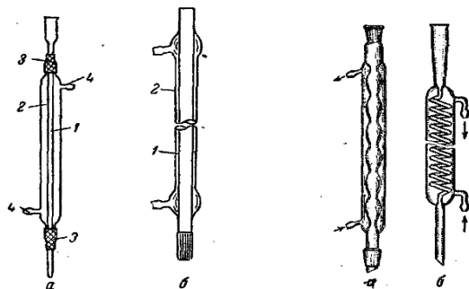
Рис. 8. А – с резиновыми муфтами; б – со шлифом; 1 – форштос; 2 – рубашка; 3 – соединительные резиновые трубки (муфты); 4 – отростки.
