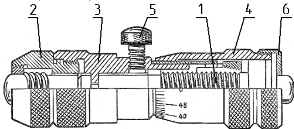
Рисунок 5.1 - Микрометрический нутромер (заполнить наименование позиций)
