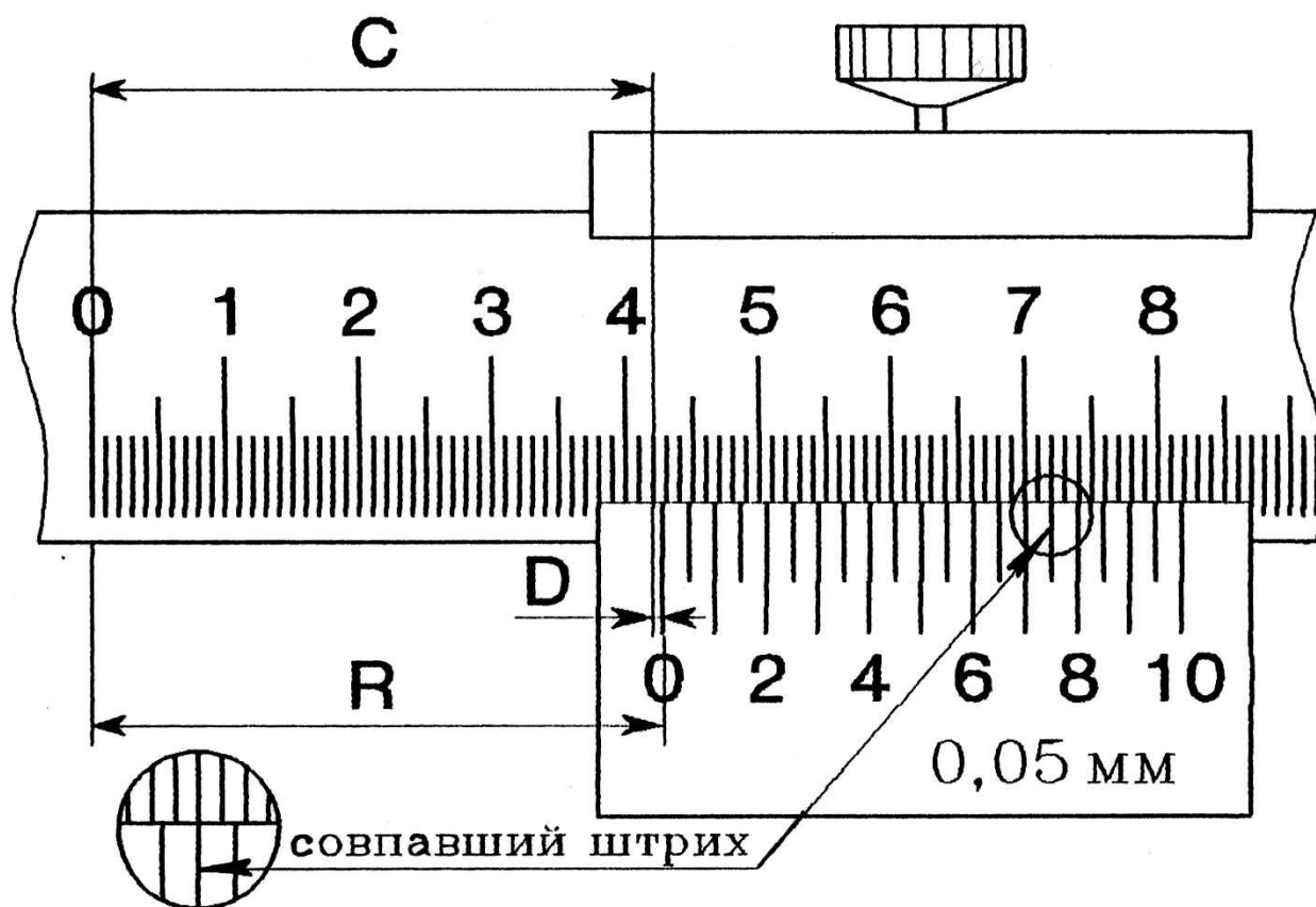
Рисунок 1.2 – Считывание показаний со штангенинструмента Порядок считывания показаний _____ (записать правило) _____ _____
