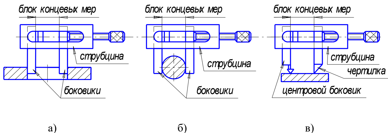
Рисунок 3.2 - Приспособления для плоскопараллельных концевых мер длины
