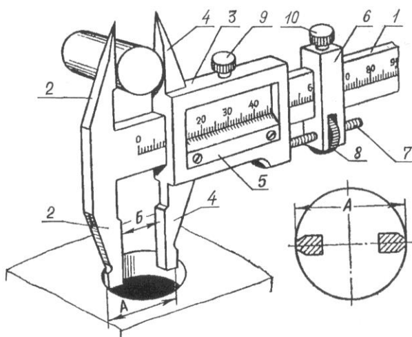
Рисунок 1.1 – Устройство штангенциркуля
